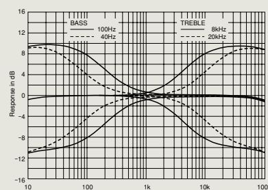
トーン・コントロール特性
