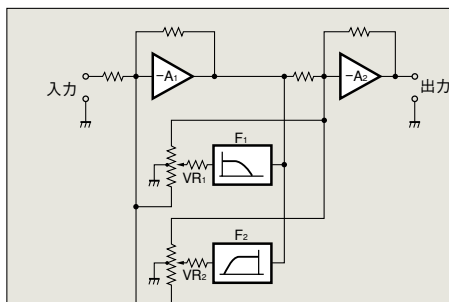
トーン・コントロール回路の原理図 (加算型アクティブ・フィルター方式)
