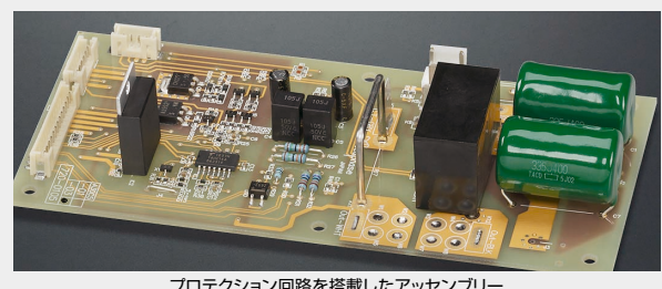
プロテクション回路を搭載したアッセンブリー
