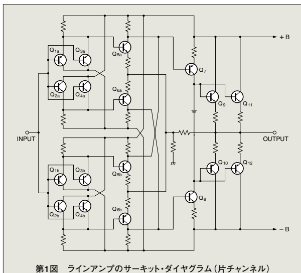
第1図 ラインアンプのサーキット・ダイアグラム (片チャンネル)
