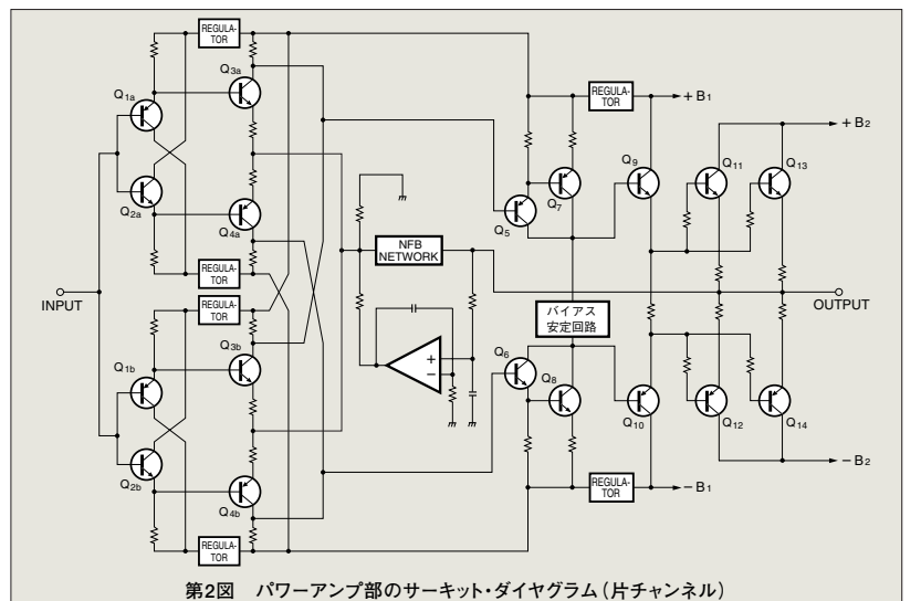
第2図 パワーアンプ部のサーキット・ダイアグラム (片チャンネル)
