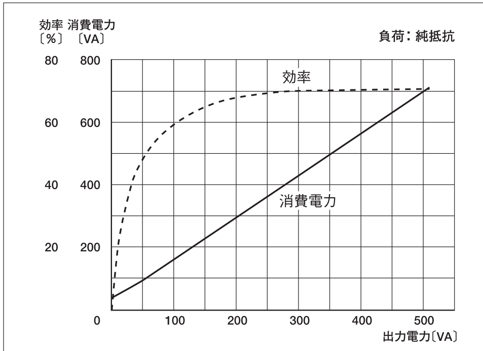
出力電力／効率・消費電力 特性図
